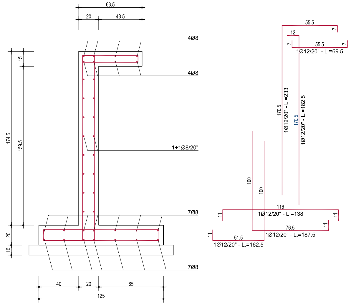
SEZIONE TRASVERSALE 1:20
