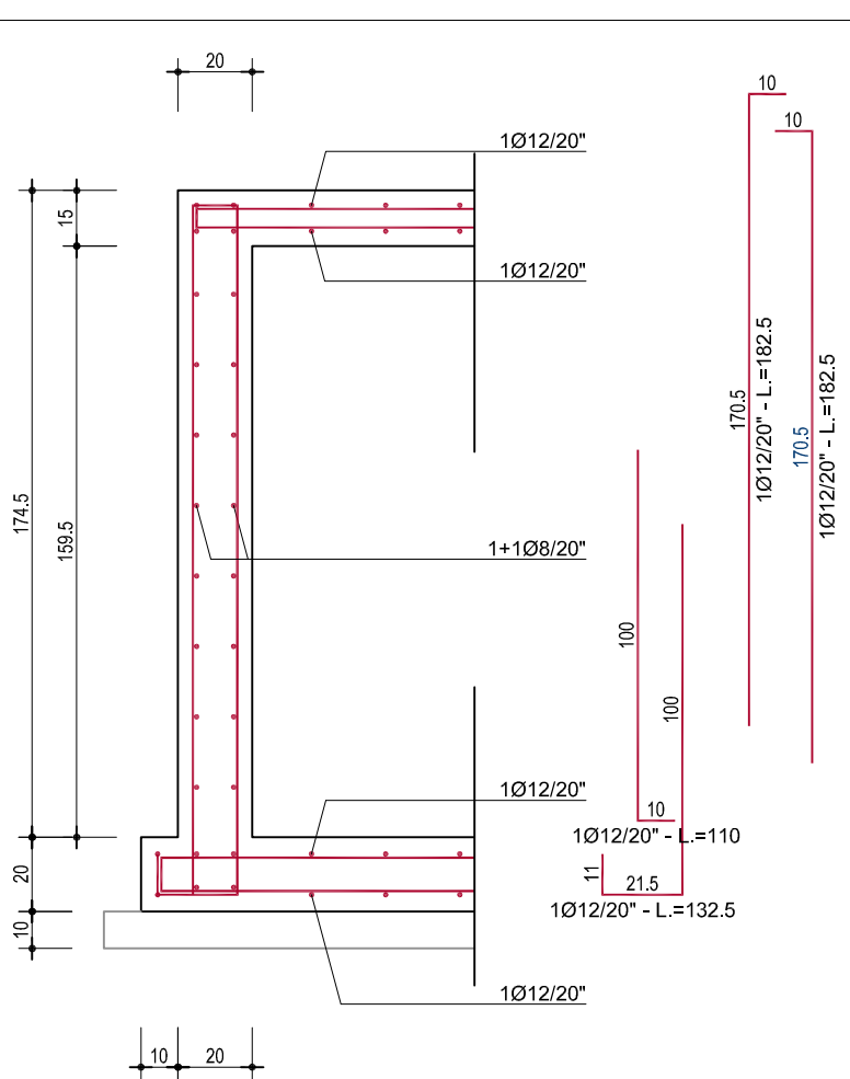
SEZIONE LONGITUDINALE 1:20
